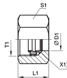
X1) 卡套
