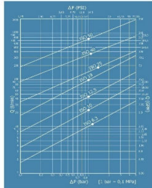
流量图
