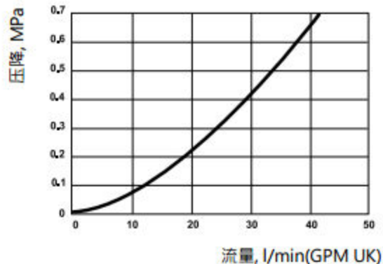
压降图
