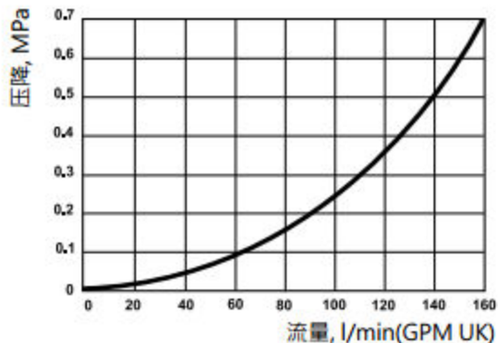
压降图
