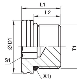
X1) O型圈
